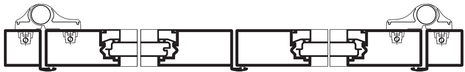
Secção B-B
