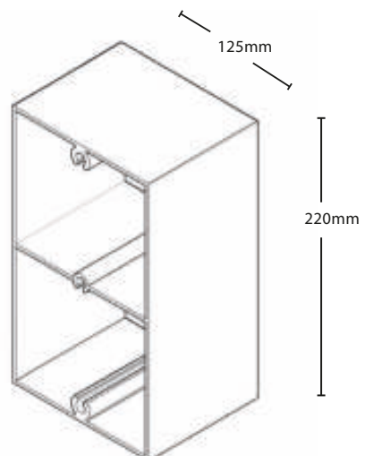
Sección Viga Travesaño
