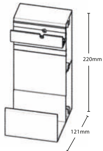
Sección Viga Canal
