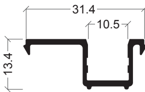
BE-11 Compensador
