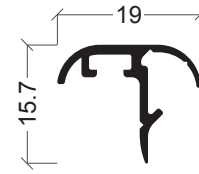
XP-04 Perfil de batente
