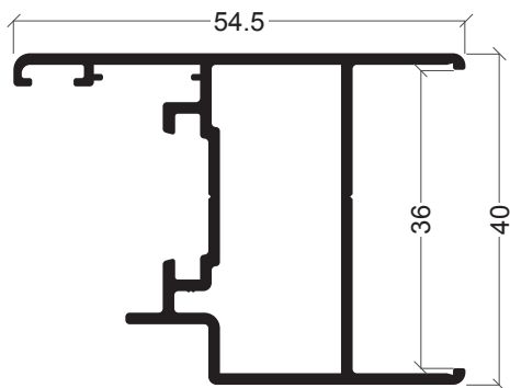
BE-02 Aro móvel caixa 36 mm
