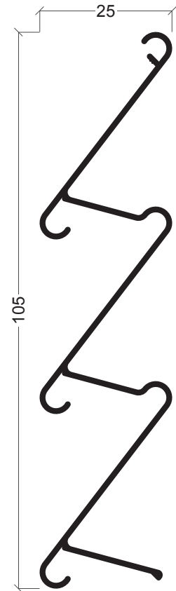
Z-20 Lâmina fixa
