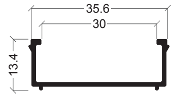
BE-14 Redutor
