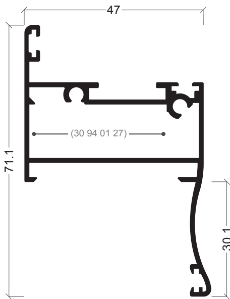
XP-09 Aro fixo com remate
