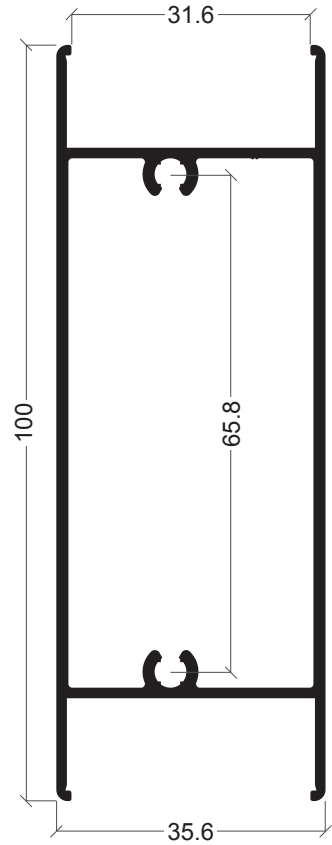
BE-10 Travessa caixa 31.6 mm
