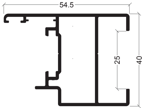
BE-19 Aro móvel caixa 25 mm
