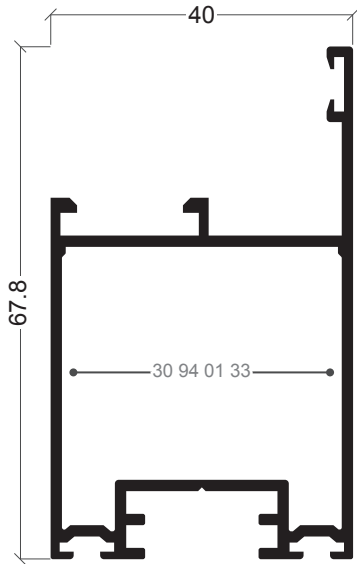
XP-22 Aro móvel com bite
