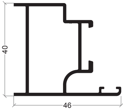
BE-01 Aro fixo
