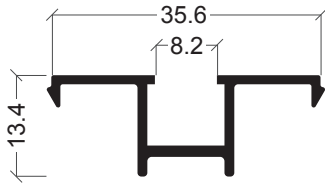
BE-07 Compensador
