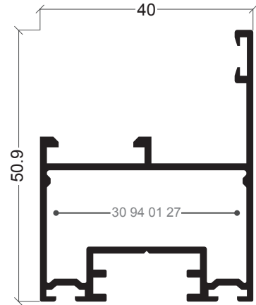
XP-11 Aro móvel com bite
