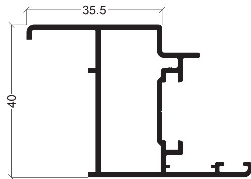
BE-17 Aro fixo com remate
