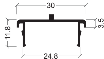
BE-18 Calha comando
