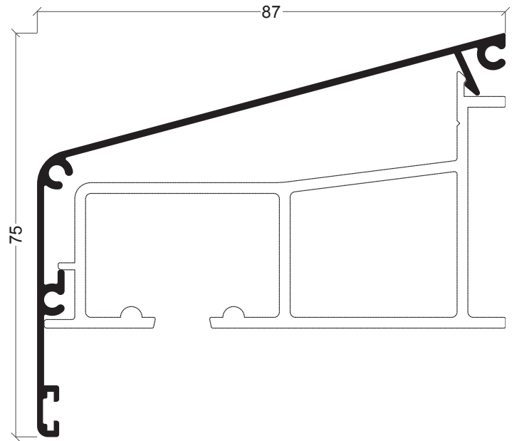
XP-12 Tampa guia superior de correr longa
