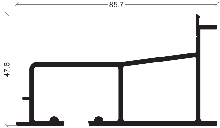
XP-13 Guia superior de correr
