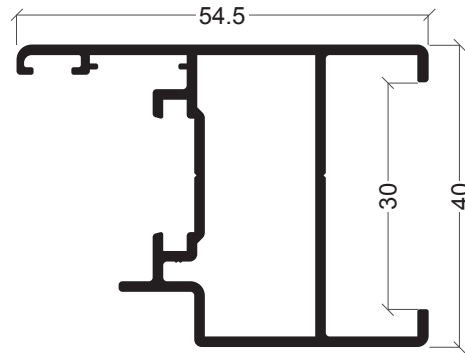
BE-03 Aro móvel caixa 30 mm
