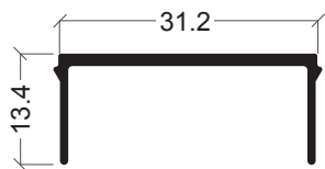
BE-12 Calha fecho
