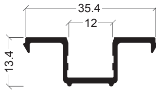
BE-15 Compensador
