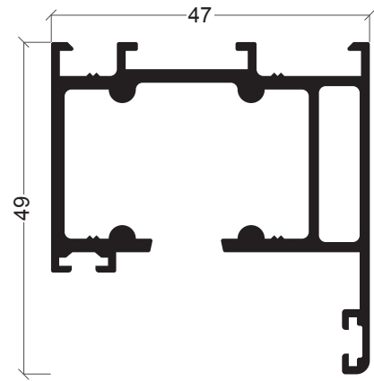
XP-21 Aro fixo de correr
