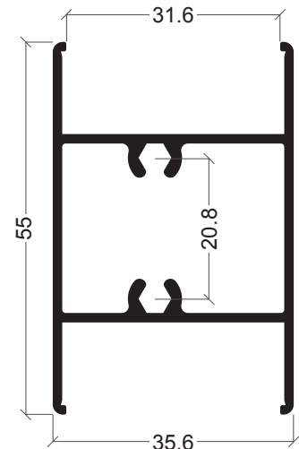
BE-06 Travessa caixa 31.6 mm
