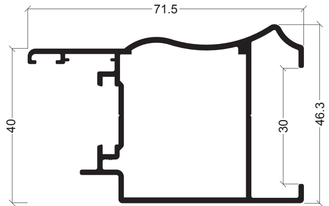
BE-24 Aro móvel decorativo caixa 36 mm
