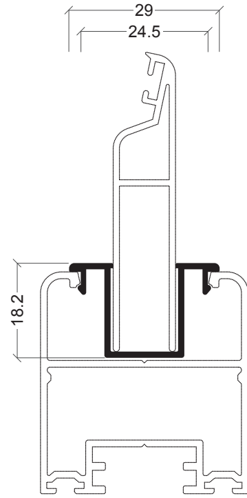
XP-19 Redutor para Z/54
