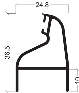
XP-02 Meia lâmina 10 mm
