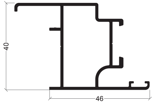
BE-27 Aro fixo com remate
