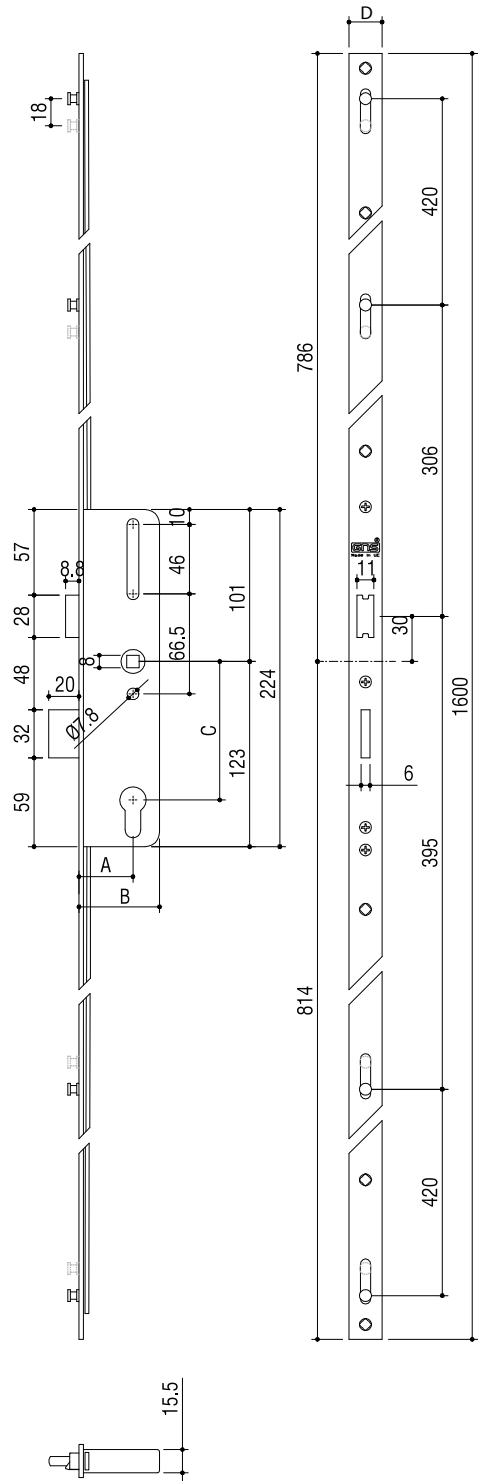
COGUMELOS/BULONES/ MUSHROOMS/ CHAMPIGNONS 5P
